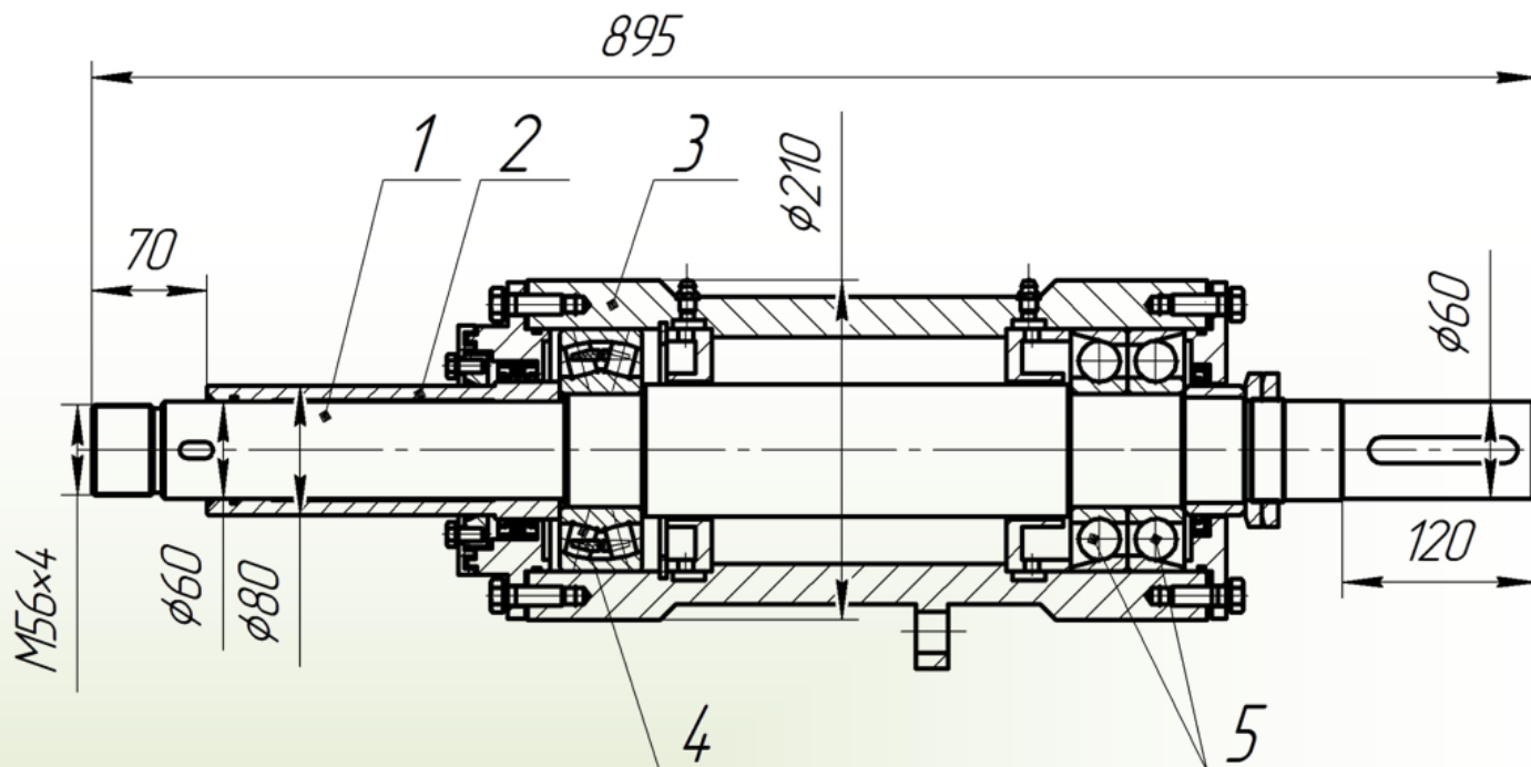
Общий подшипниковый узел в сборе (Вал в сборе, черт. № У150-30.010М-03СБ)
